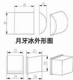
方冰外形图
