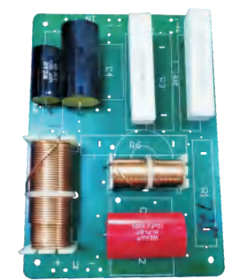
JB-1
