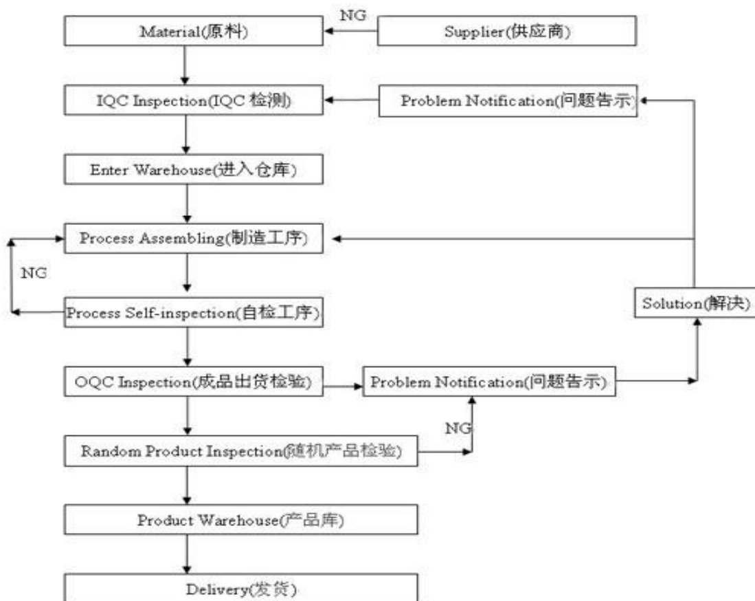
Quality Control Flowchart 质量控制流程图
