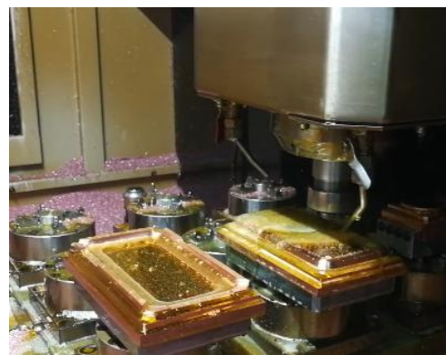
CNC processing die process CNC加工处理模具工序
