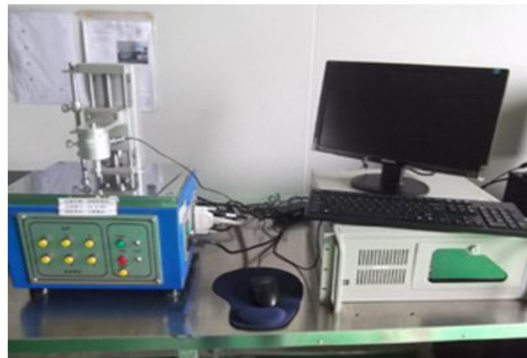
Force load tester 荷重曲线
