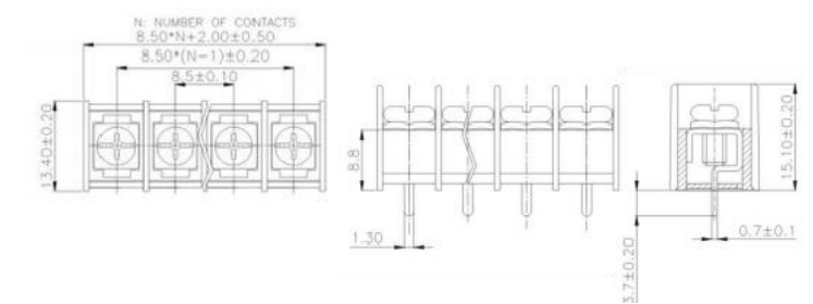
KF35C KF35CM
