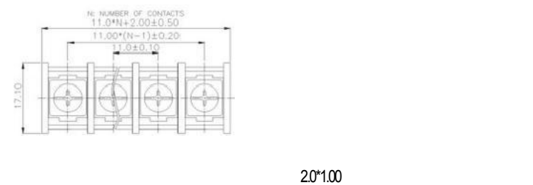
KF65C KF65CM
