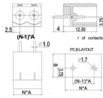
KF2EDGV
