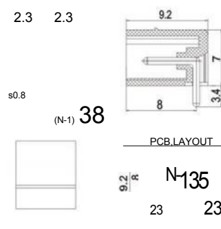
KF2EDG-3.5R KF2EDG-3.81R
