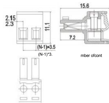
KF2EDG-3.5 KF2EDG-3.81
