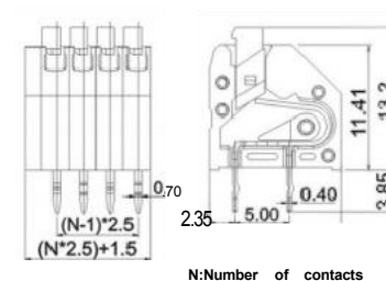
KF250B-2.5
