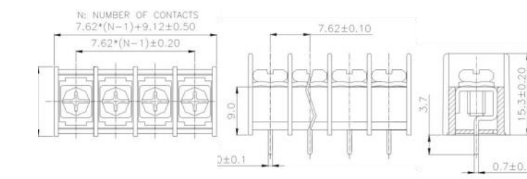
KF25C KF25CM
