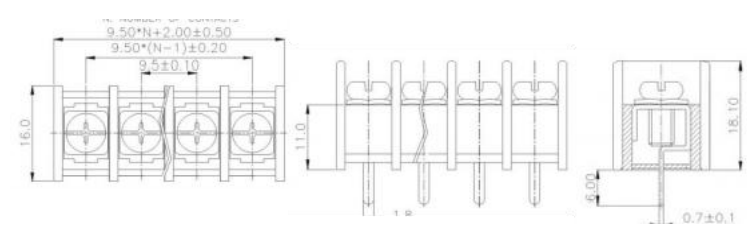
KF45C KF45CM
