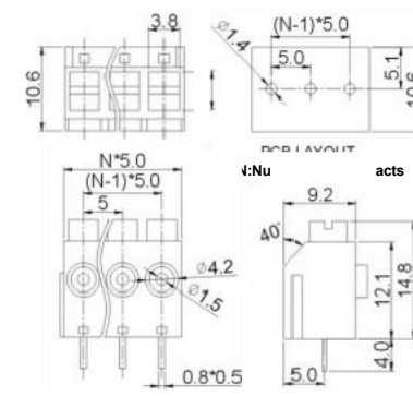
KF390
