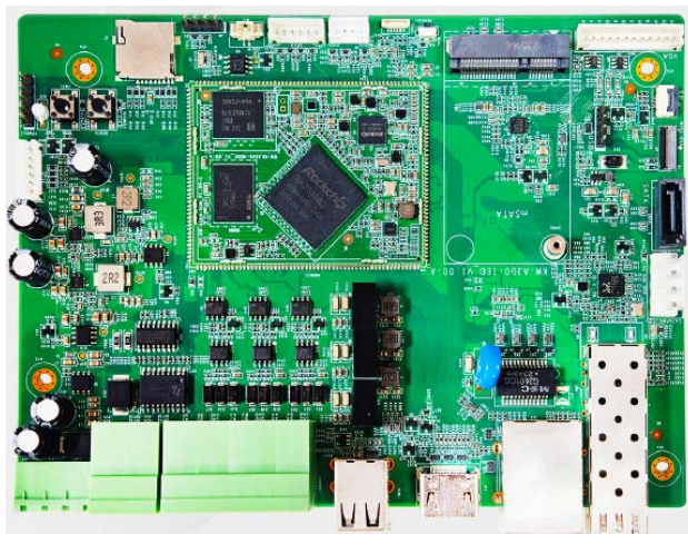
RK3588 主板
