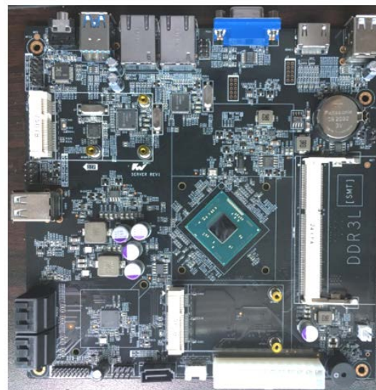
KW S100 主板 : KWHM01
