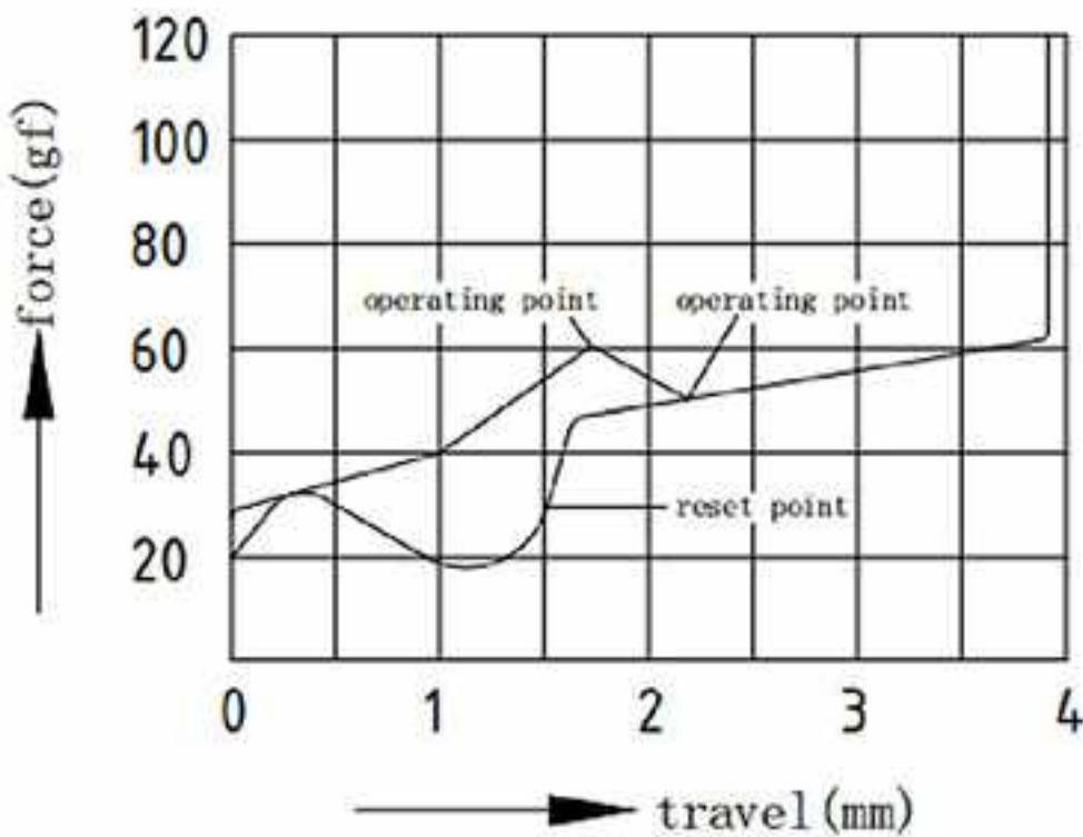
force-travel-diagram 操作力-行程-图解
