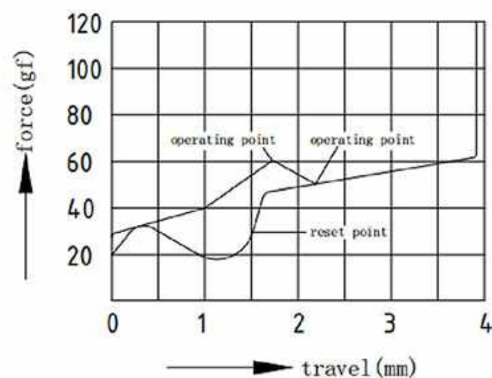
force-travel-diagram 操作力-行程-图解
