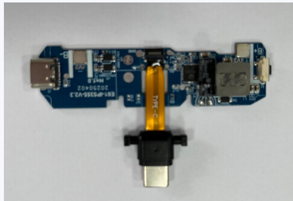
Power Bank 移动电源
