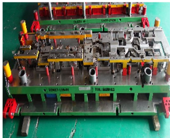
Progressive Die
