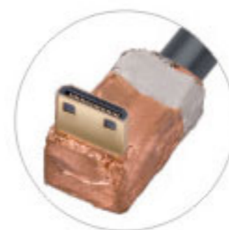
Mini HDMI Male 90° 360° Copper Foil Wrap Soldering Shield
